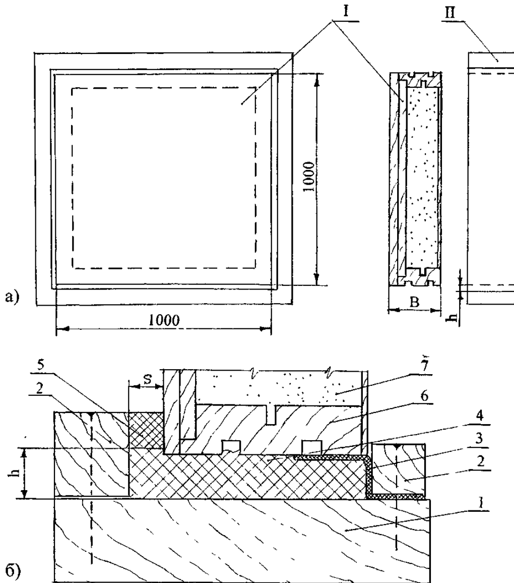
а) блок-панель з блок касетою, б) виконання з'єднувального шва I – блок-панель товщиною B , що дорівнює товщині віконного (дверного) блока; II – блок-касета для установлення блок-панелі ( h , s – зазори для з'єднувального шва)
